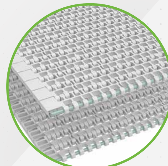
1096 Flush Grid
